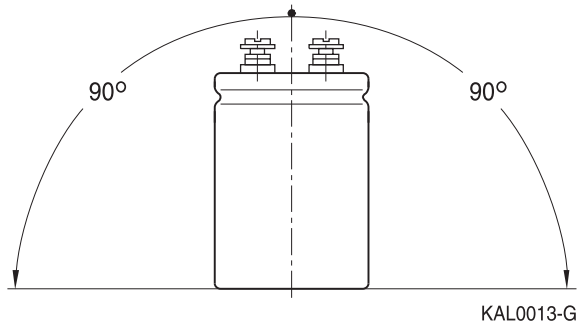
Рис. 30. Рекомендованный диапазон установочных положений
