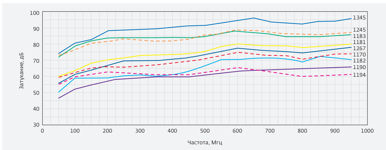
Рис.3. Эффективность экранирования (затухание в дальней зоне). Типичные величины (метод измерений ASTM-D-4935)
